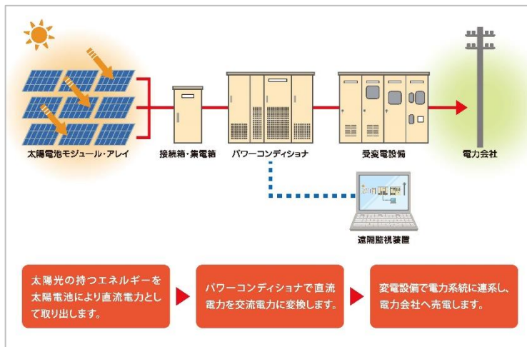
「太陽光発電所の仕組み」
