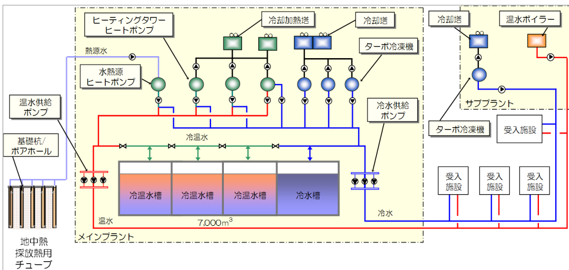
「東京スカイツリー地区熱供給施設のシステムフロー」
