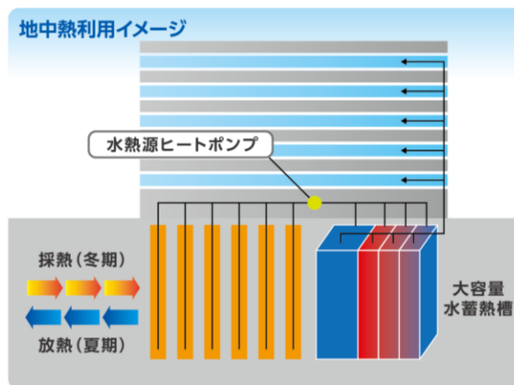
地中熱利用システム
